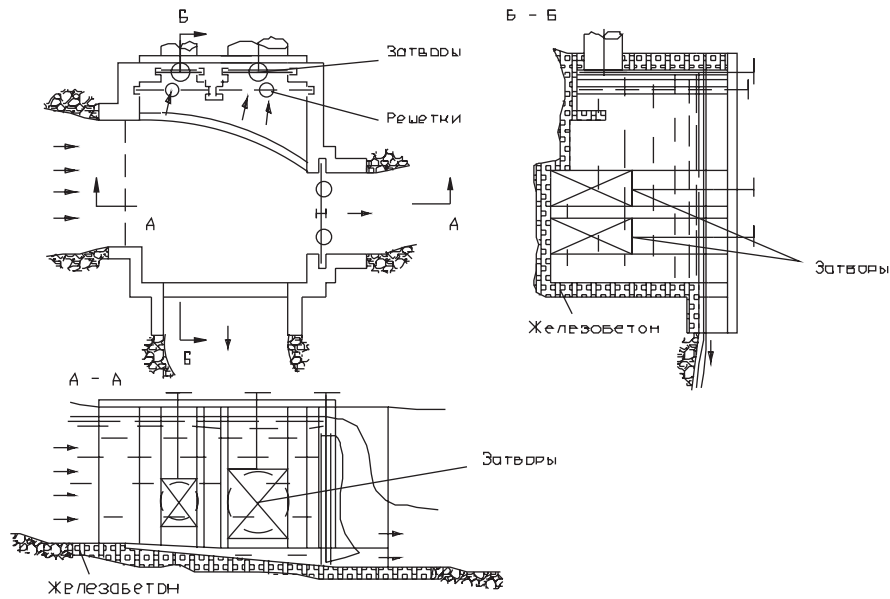
Рис. 2.3.4 Напорный бассейн
